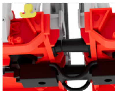
Luftleitungen zwischen den beiden Wagenhälften dargestellt und kurzgekuppelt
