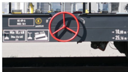
Extra angesetztes Handbremsrad
