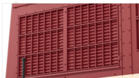
Lüfterjalousie Vorbildgerecht je nach Bauserie ausgeführt
